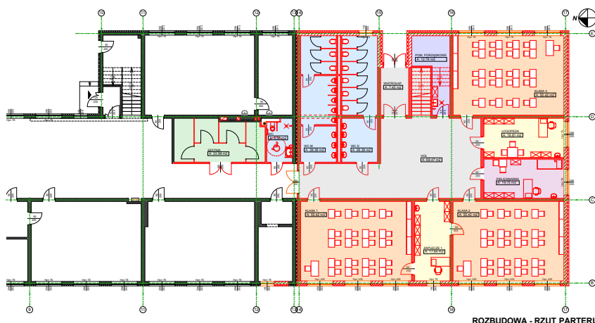
ROZBUDOWA - RZUT PARTERU
