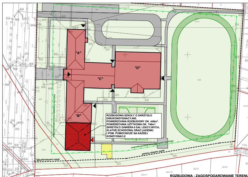
ROZBUDOWA - ZAGOSPODAROWANIE TERENU
